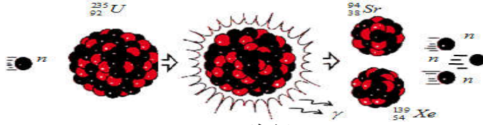
انشطار نووي
