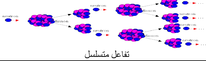
انشطار نووي
