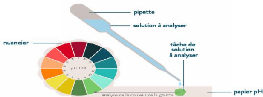
Estimation du pH à l'aide d'un papier pH
