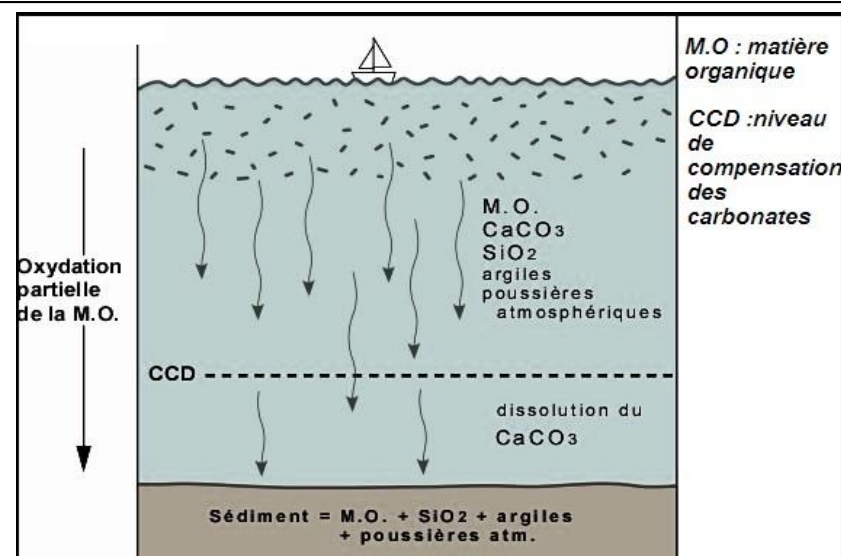
Figure 3 : Conditions de sédimentation de calcaire, de silice et de l'argile
