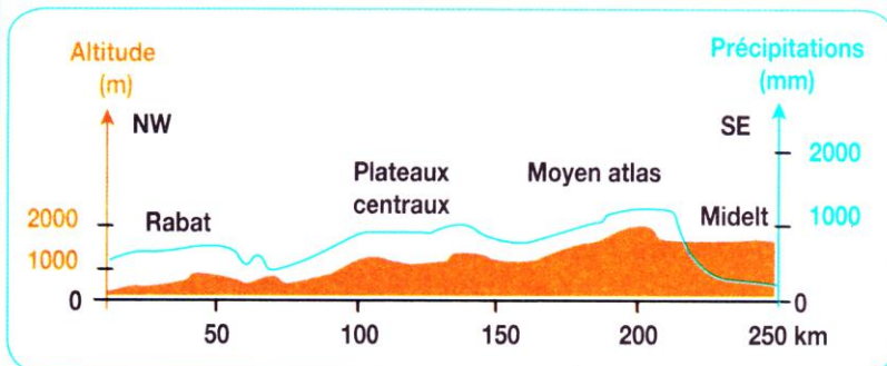
Figure 5 : Évolution des précipitations annuelles selon la topographie
