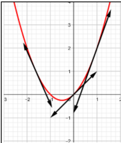
Graphe d'une fonction convexe
