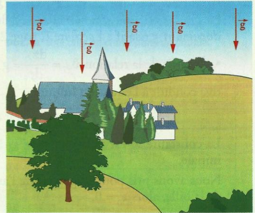
Doc. 7 Sur des distances horizontales et sur des hauteurs de quelques kilomètres, on peut admettre que le champ \vec{g} est uniforme.
