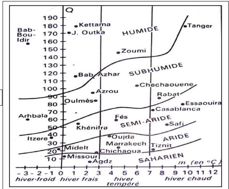
Document 1 : Diagramme d'Emberger
