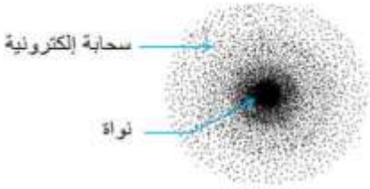
النموذج الحالي (شرودينجر و دوبروكلي)
