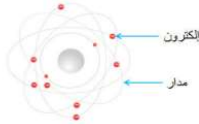
نموذج سابق للذرة (بوهر و بيزان)
