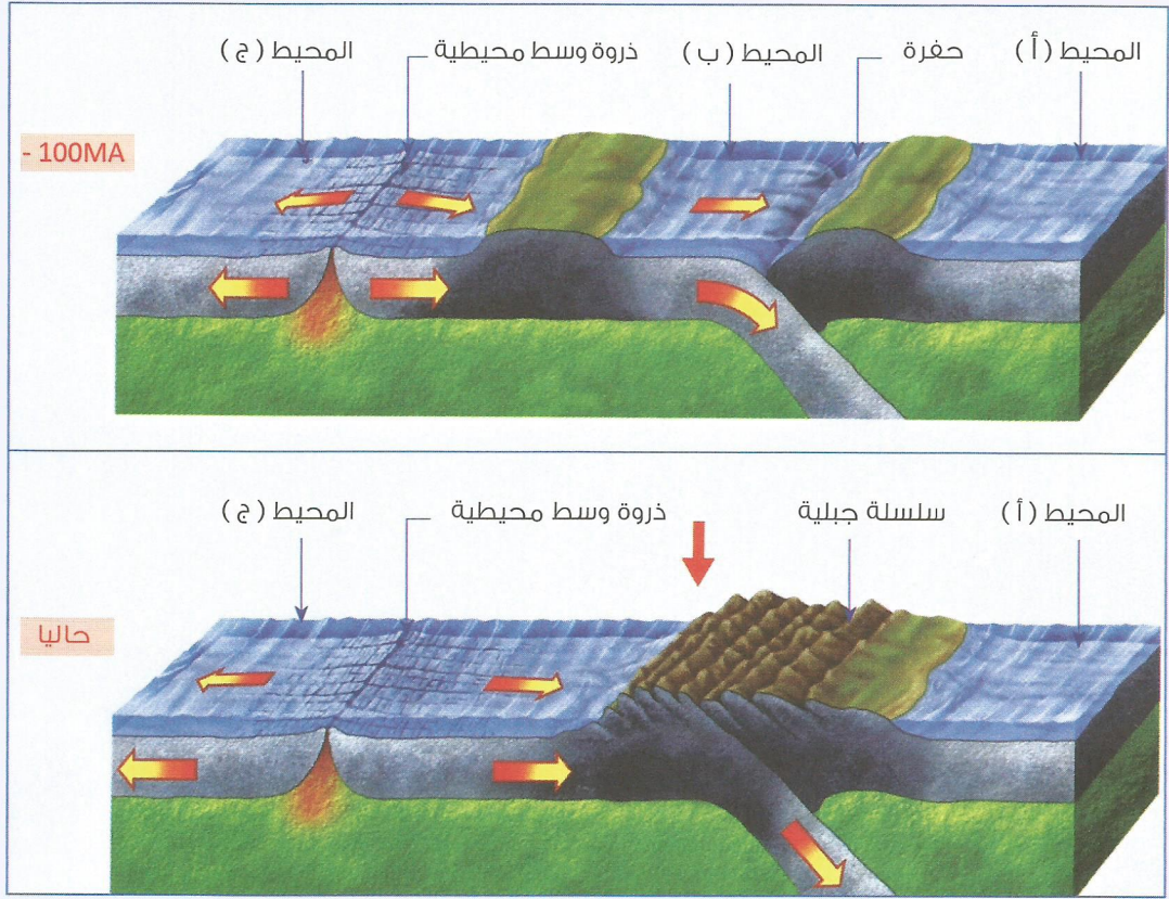
سلاسل الطمر – Chaîne de subduction
