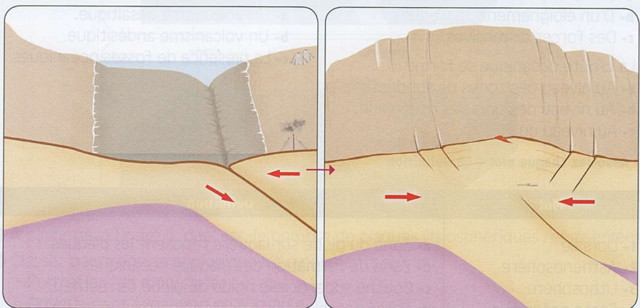
Convergence de palques, fermeture d'un océan et formation d'une chaîne de collision
