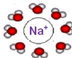
hydratation de l'ion \text{Na}^+
