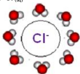
hydratation de l'ion \text{Cl}^-
